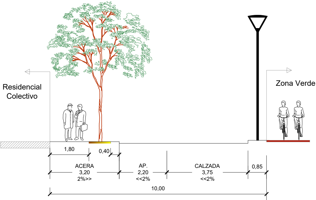
SECCIÓN 1.1 EJES: 15
