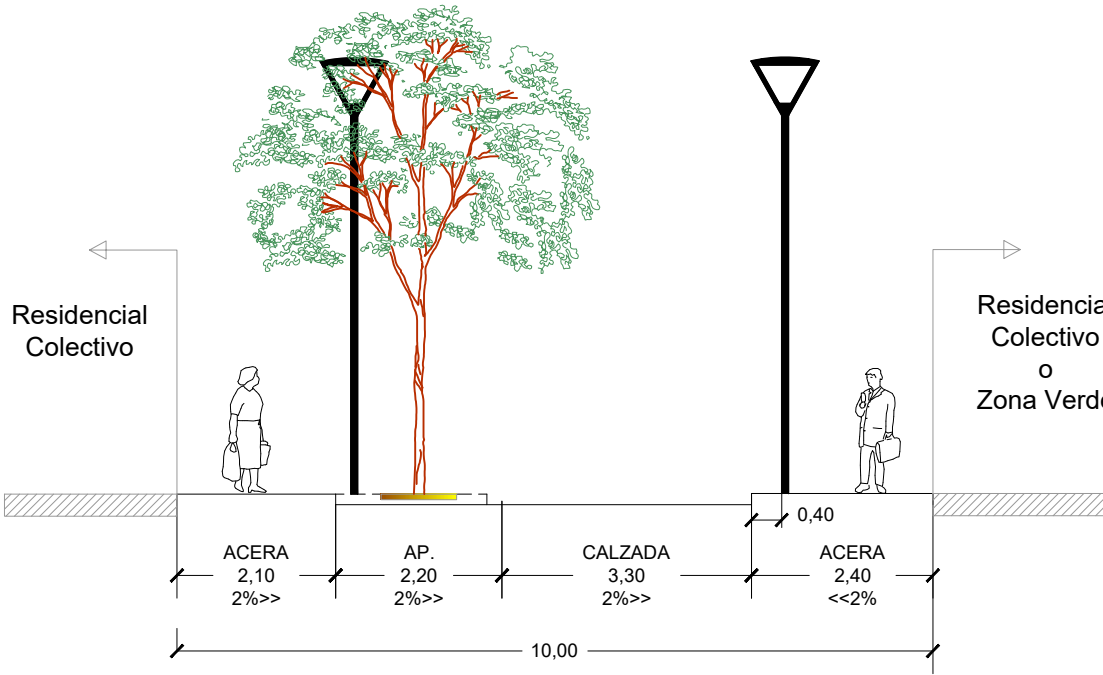
SECCIÓN 1.2 EJES: 9 / 10
