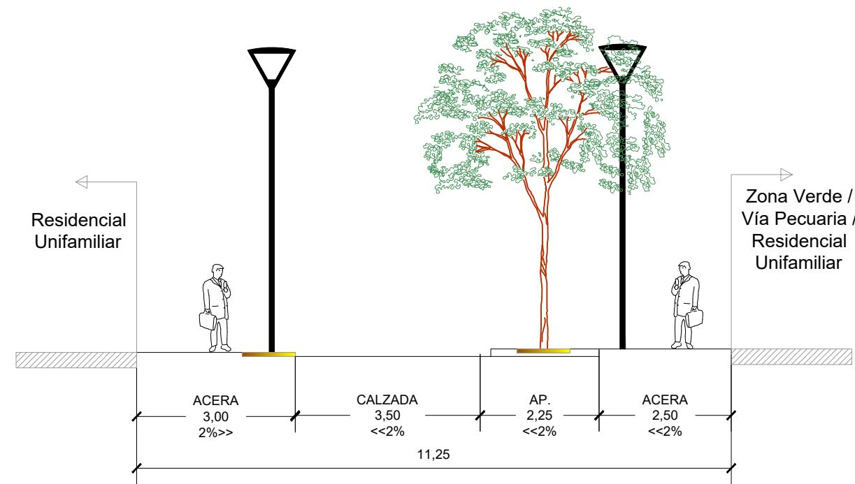
SECCIÓN 2.1 EJES: 57 / 58 / 59 / 60 / 69 / 70
