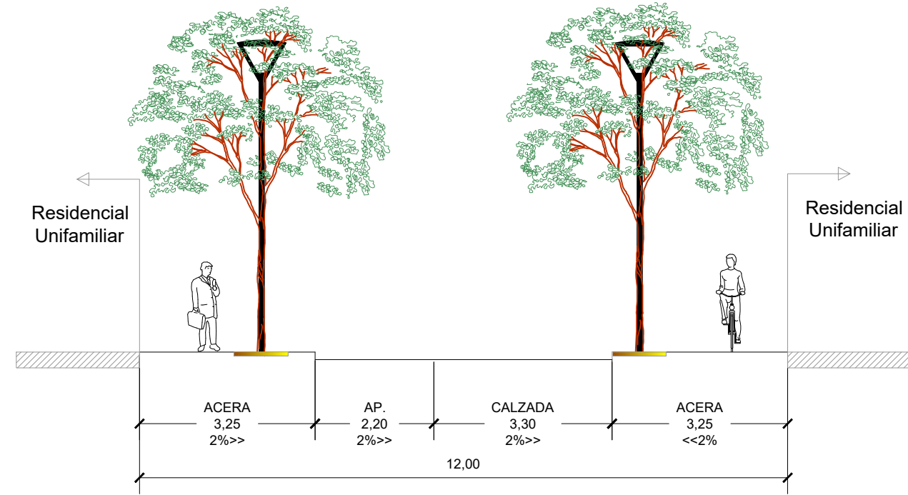
SECCIÓN 2.2 EJES: 81
